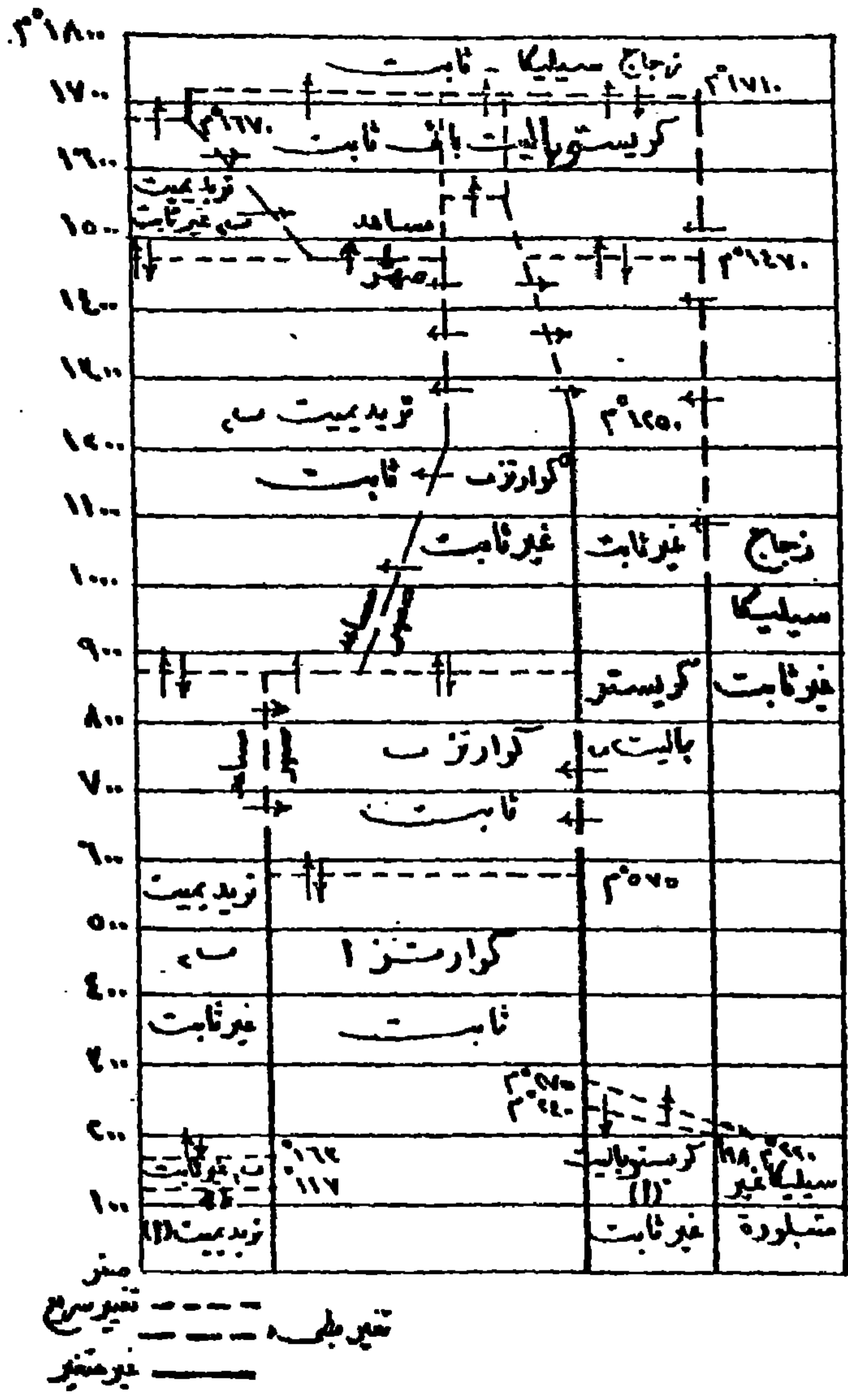
(شكل رقم ١) التآصل البلوري بين معادن السيليك
